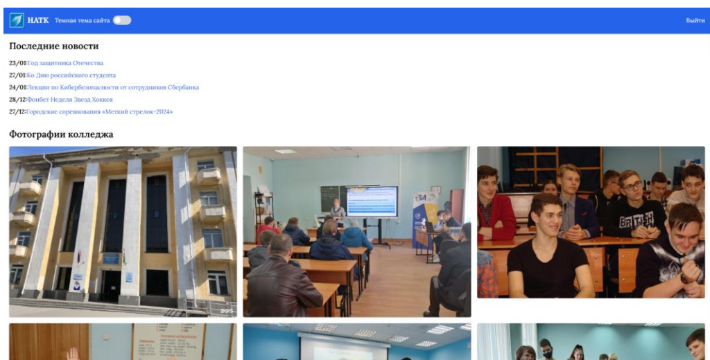
Рисунок 2 – Главная страница
