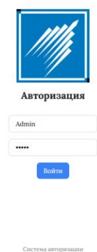
Рисунок 1- Страница авторизации
